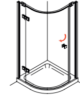
Argos WP 265 Viertelkreis-Dusche mit einer Drehtür
