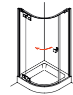
Triton WP 230 Pendeltür am Fixteil mit Seitenwand
