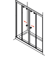
Poseidon 375 Doppel-Schiebetür in Nische
