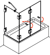
Neptun 480 Falttür mit Seitenwand auf Badewanne
