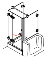
Proteus WW 234 U-Kabine mit Drehtür und verkürzter Seitenwand
