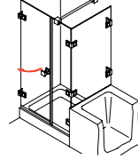
Argos WW 141 Drehtür und Fixteil mit verkürzter Seitenwand
