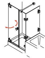
Triton WW 141 Pendeltür und Fixteil mit verkürzter Seitenwand
