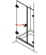
Argos WW 110 Drehtür und Fixteil in Nische
