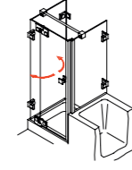
Triton WW 234 U-Kabine mit Pendeltür und verkürzter Seitenwand
